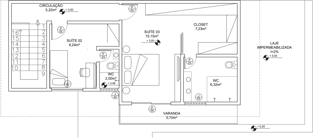
PLANTA BAIXA SUPERIOR
