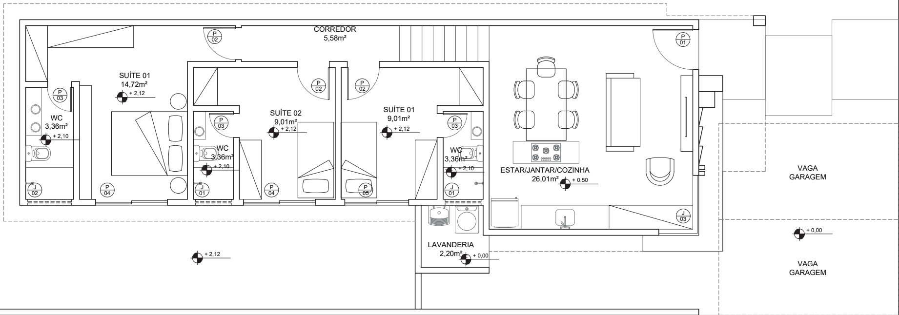
PLANTA BAIXA TÉRREO
